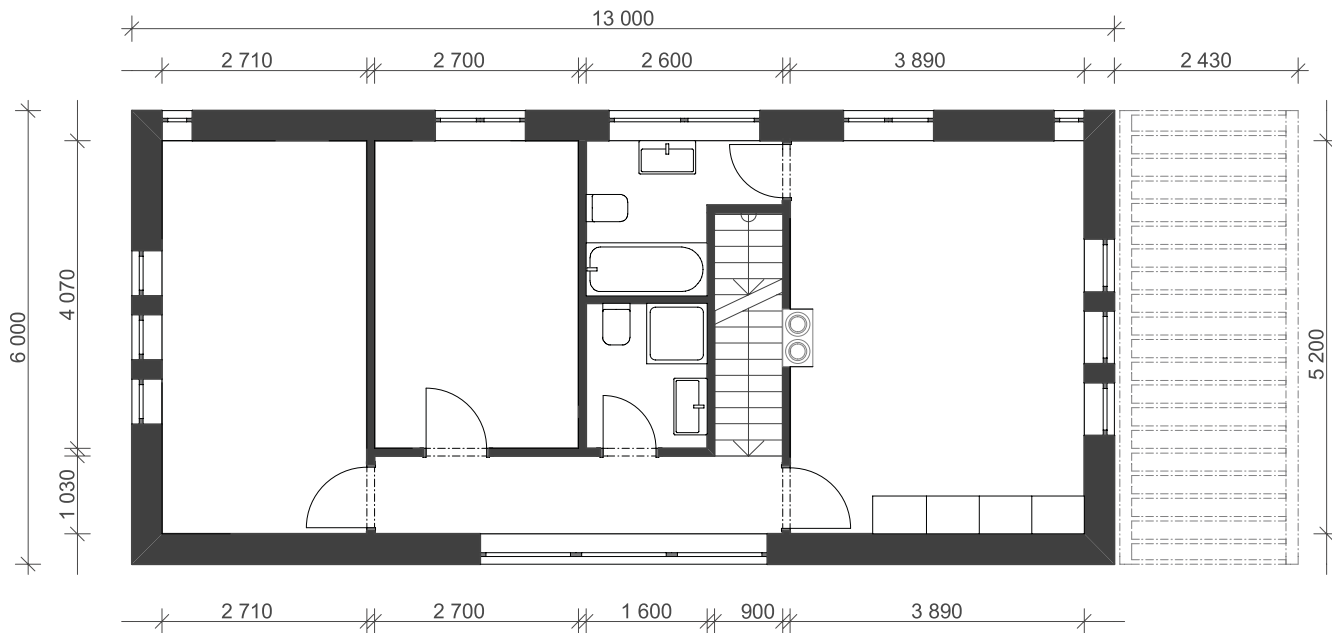
PÔDORYS 2.NP
