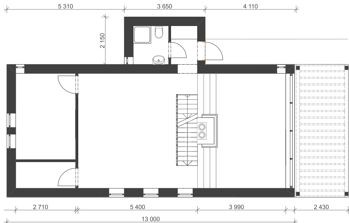
PÔDORYS 1.NP
